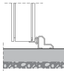
Plaatsing op de afgewerkte vloer. Er is sprake van een dorpel.
