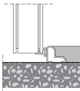
Plaatsing op de ruwe betonvloer. De vloerafwerking wordt achteraf aangebracht
